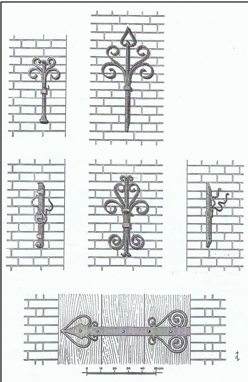
Zieranker und Zierhänge im Kreis Tondern, aus: Denkmäler des alten Bauhandwerks in Schles- wig-Holstein
